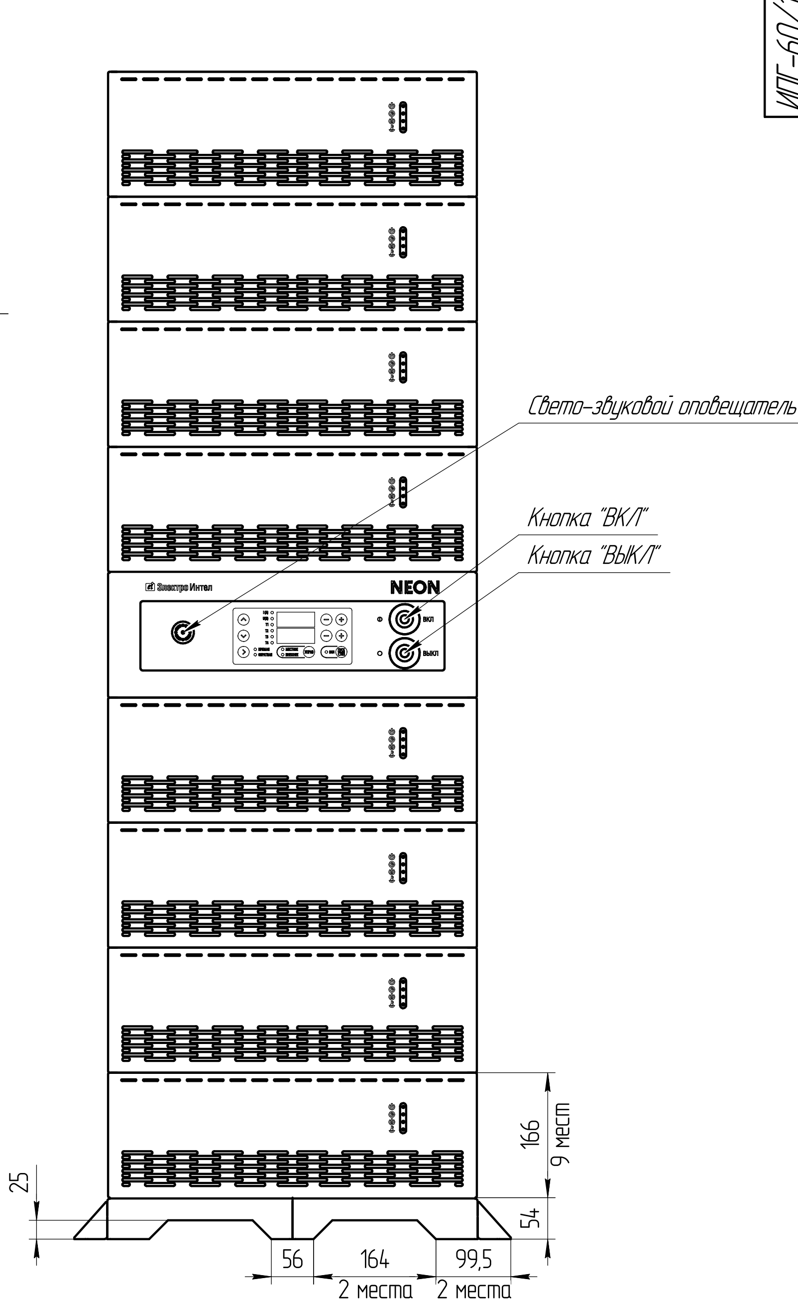
Вид спереди
