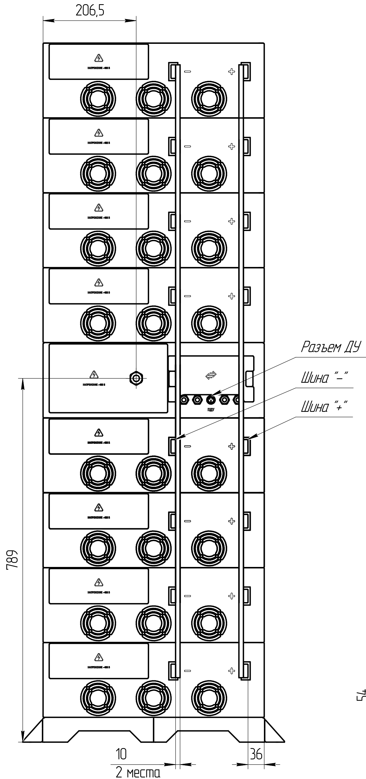
Вид сзади
