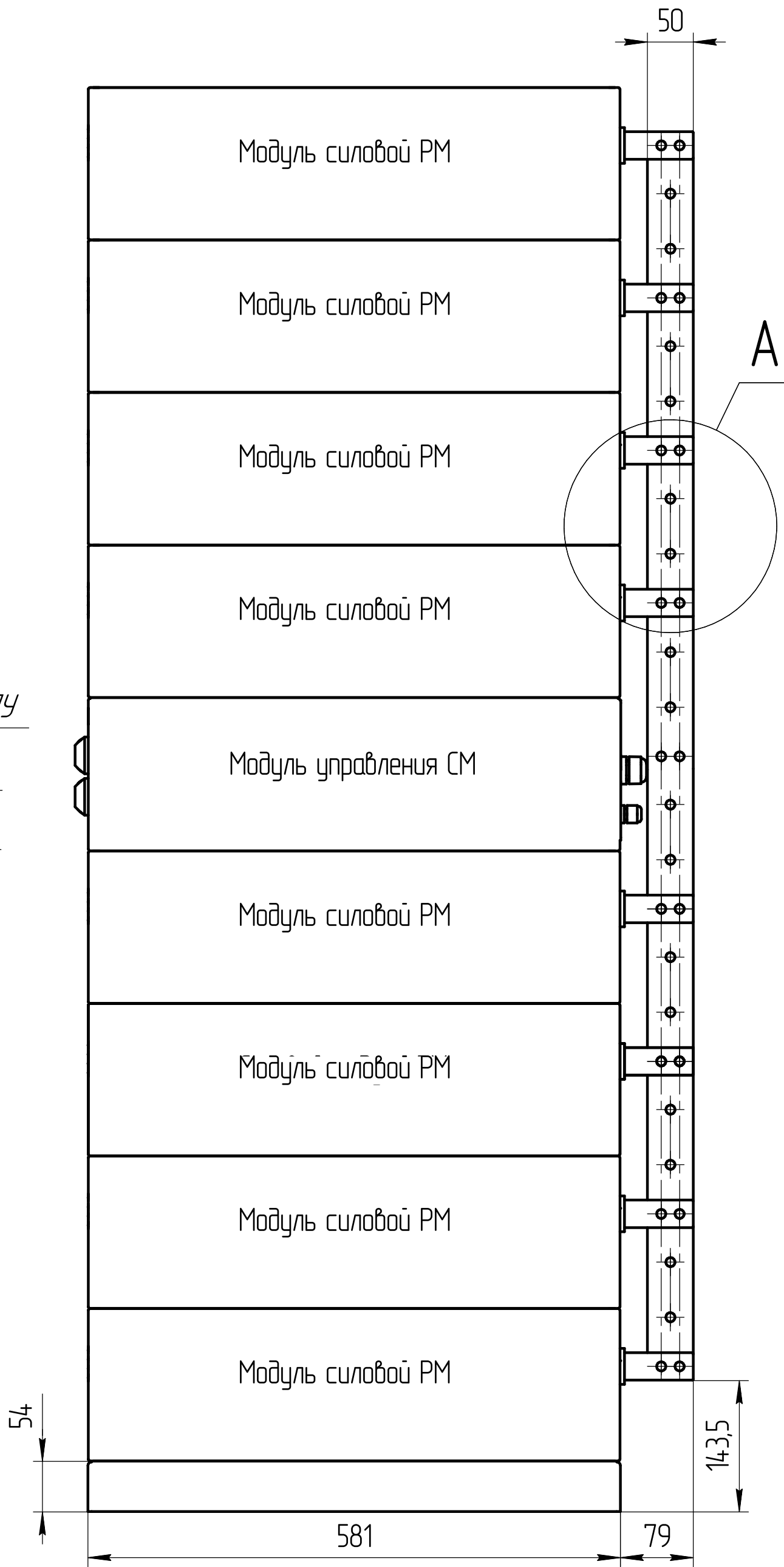
Вид сбоку
