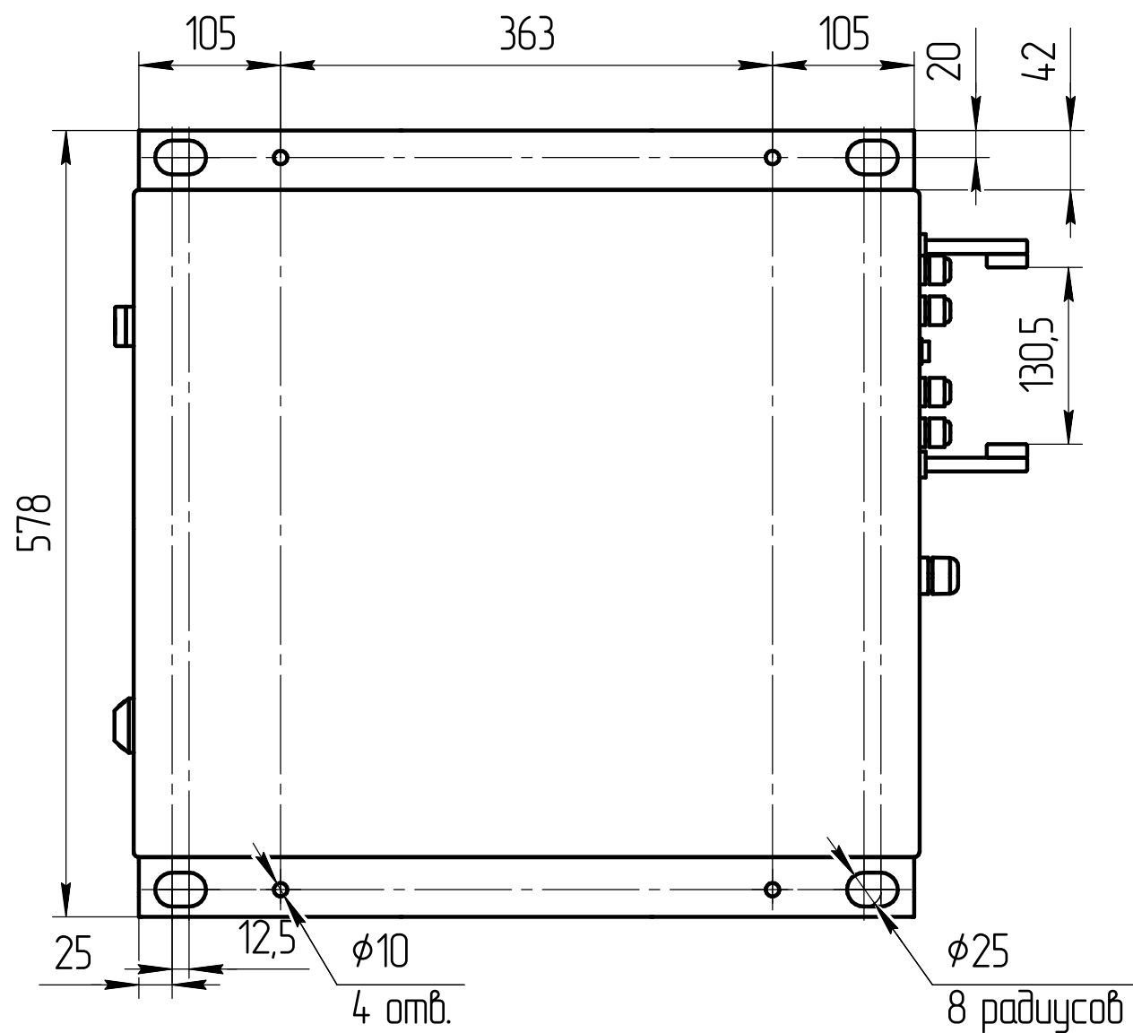
Вид сверху
