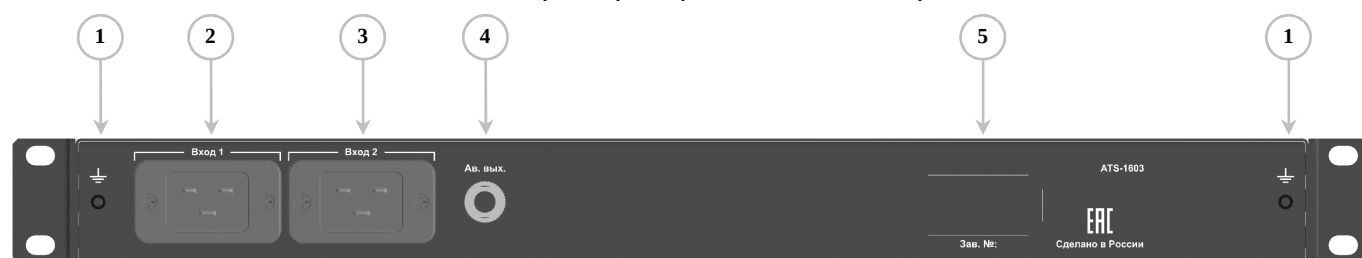
Рисунок 2 – Электронно-механический АБР ATS-1603, задняя панель:
